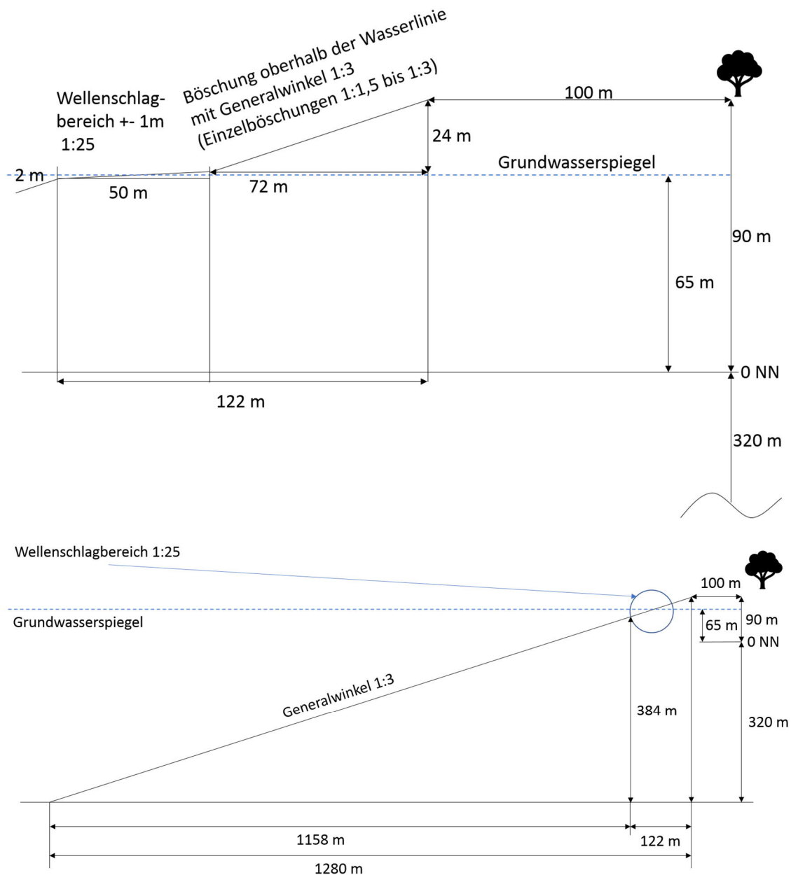
Abbildung 7: Tagebau Hambach, Gewinnungsböschung 1:3, östliche Böschung im Bereich Manheim
