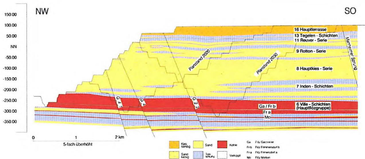
Abbildung 10: Längsschnitt 10 Tagebau Hambach NW – SO
