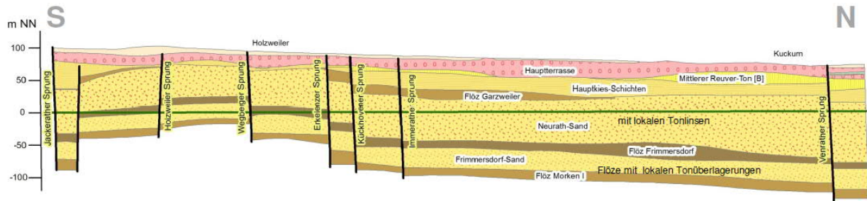
Abbildung 15: Geologischer Schnitt Garzweiler, Kuckum bis Holzweiler
